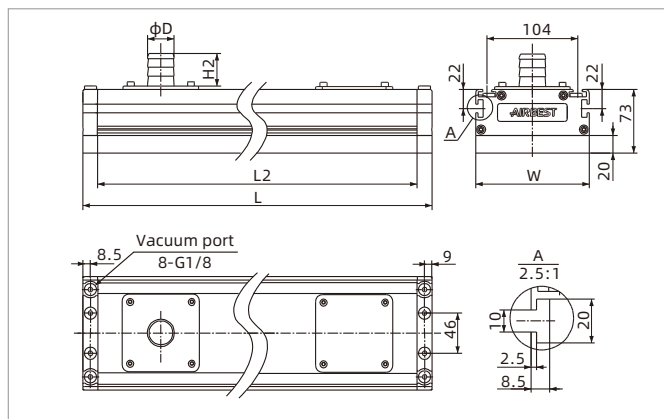
TXM130×400(600-1400)-A Sponge type
